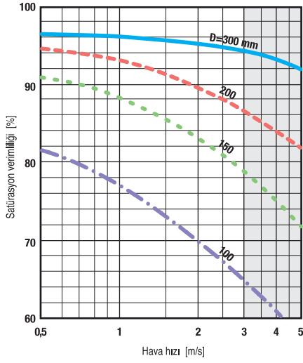
Satürasyon verimliliği CELdek 7090-15
