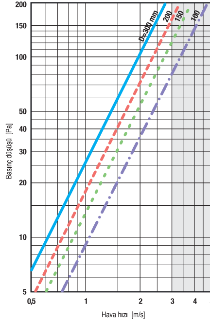
Basınç düşüşü CELdek 7090-15
